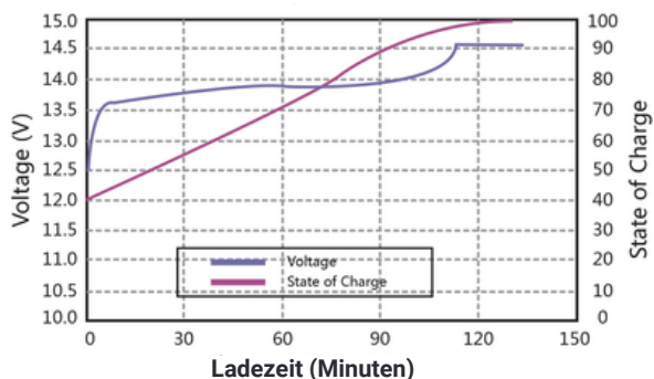
Ladezustands-Kurve @0,5C 25°C
